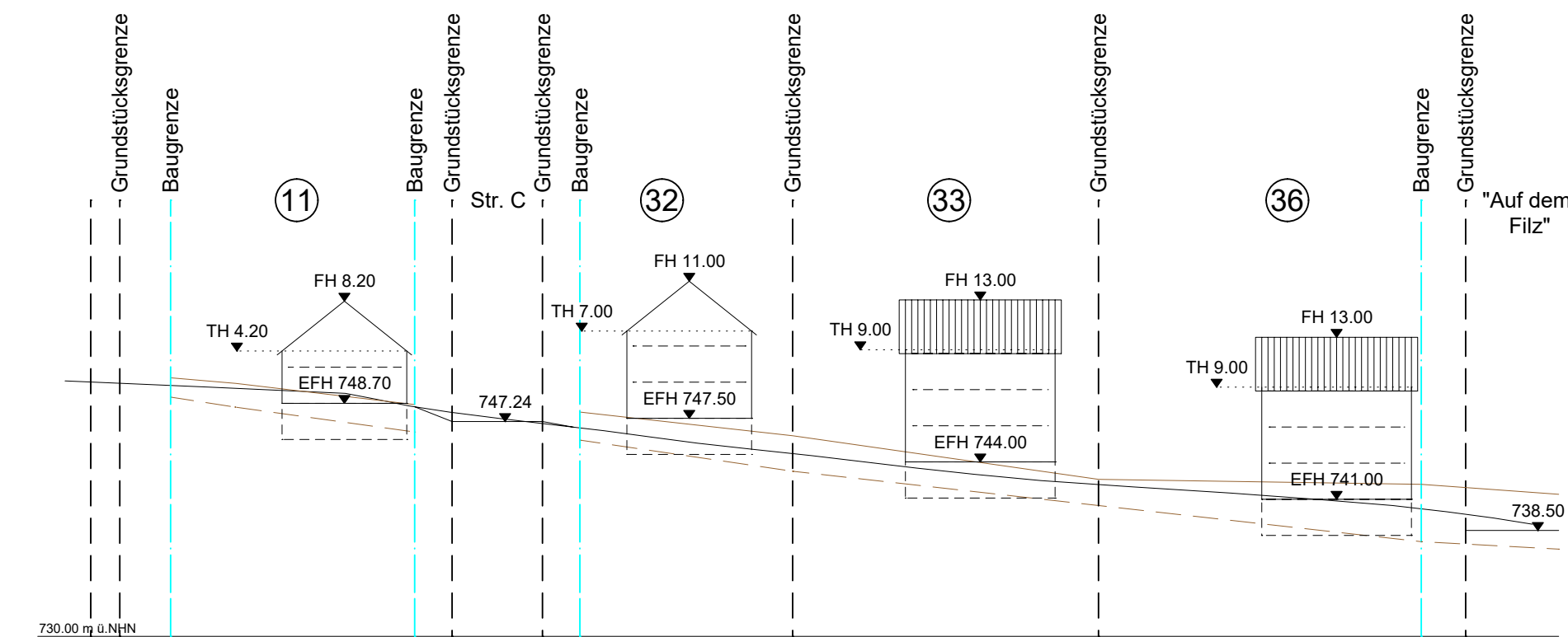
Geländeschnitt - Blickrichtung Nord
